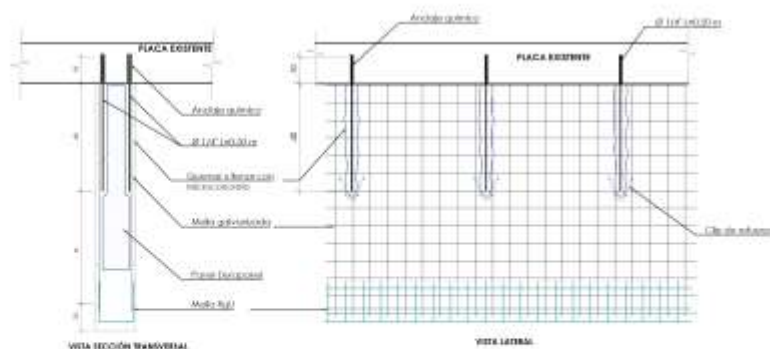
DETALLE DE CUELGA DURAPANEL CON VIGA EN CONCRETO
