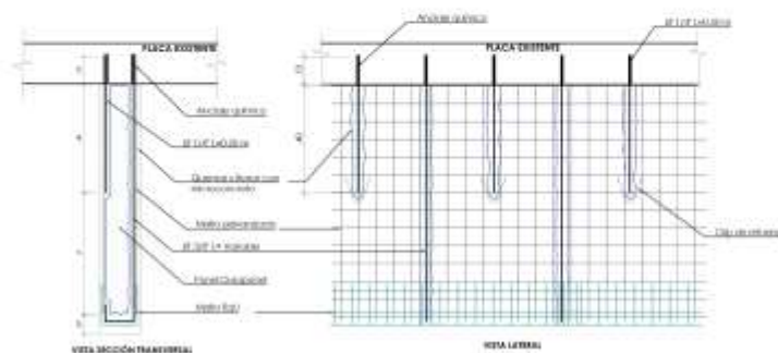
DETALLE DE CUELGA DURAPANEL CON REFUERZO ADICIONAL EN GANCHO
