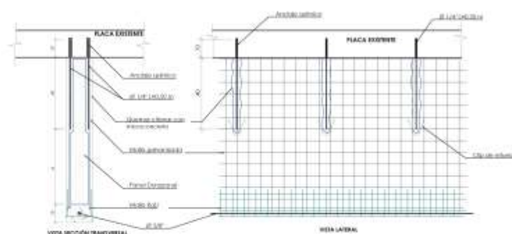
DETALLE DE CUELGA DURAPANEL CON REFUERZO ADICIONAL
