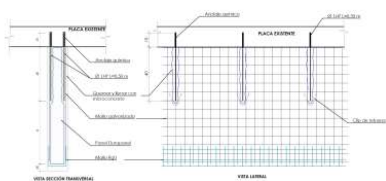
DETALLE DE CUELGA DURAPANEL
